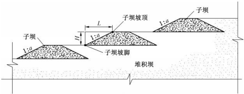
图 3-2 堆积子坝外坡比计算示意图
